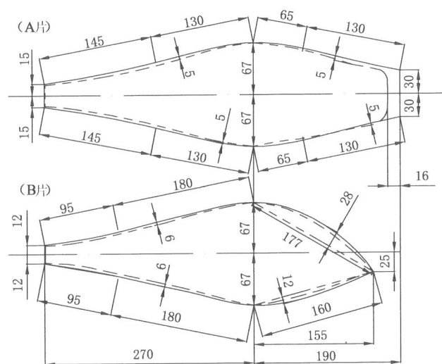
图 F.4 皮革袋 A 片和 B 片示意图
