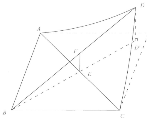
图 13 扭曲测量示意图
