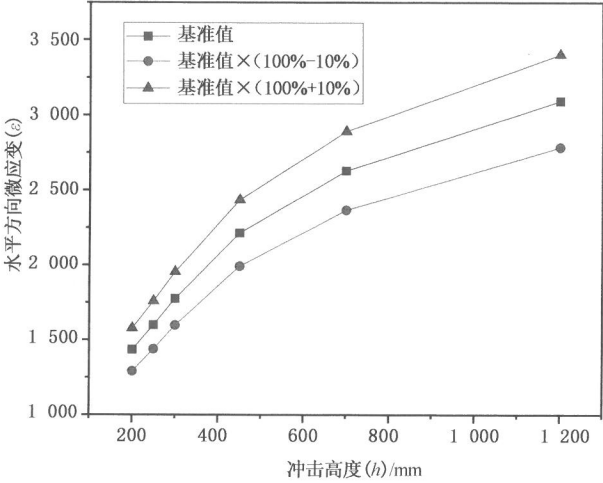
a) 霰弹袋冲击试验水平微应变基准值曲线图
