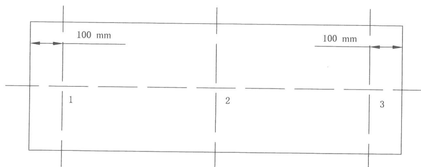
图 16 短边长度不小于 300 mm 的钢化玻璃测量点示意图
